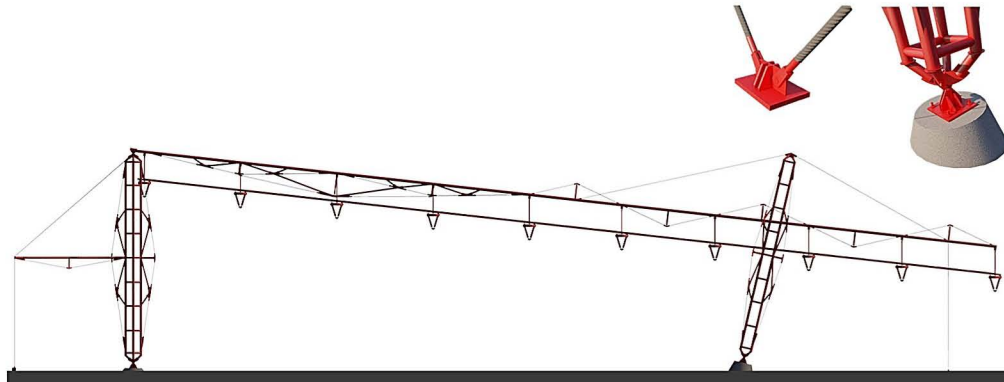
نمای شرقی سازه ای
