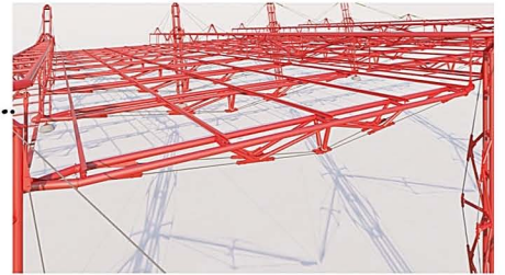
دیتیل سازه ای: تیرچه
