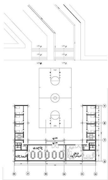
پلان واحد اقامتی
