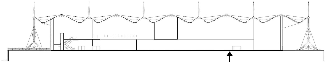
Section A-A Scale 1:200
