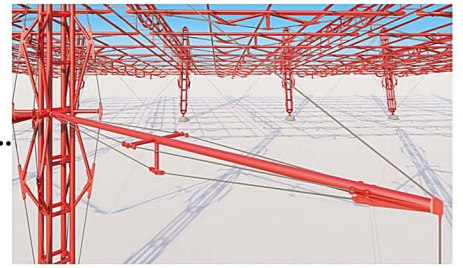
دیتیل سازه ای: تیر فرعی
