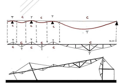
طراحی تیر و ستون مدولار بر پر اساس تنش
