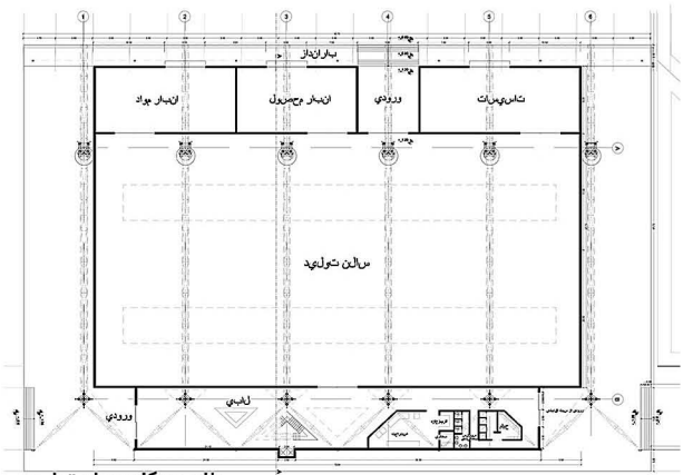
پلان همگف سوله تولید
