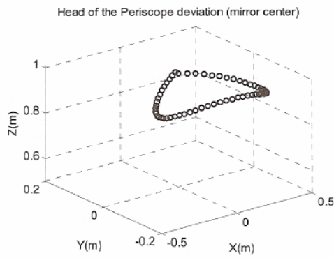
شکل ۱۴: حرکت قسمت انتهایی پریسکوپ در مختصات دکارتی
