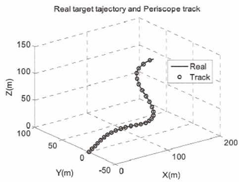
شکل ۱۶: با پایدارسازی
