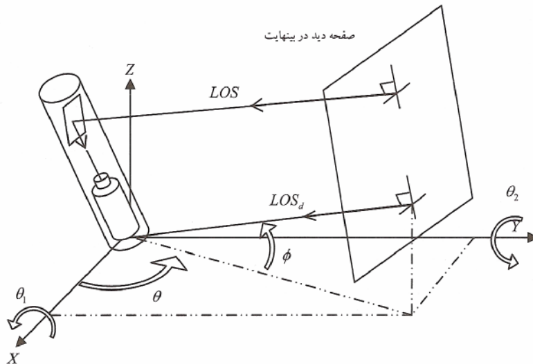
شکل ۸: صفحه دید، خط دید مطلوب و واقعی
