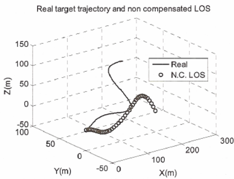
شکل ۱۵: بدون پایدارسازی
