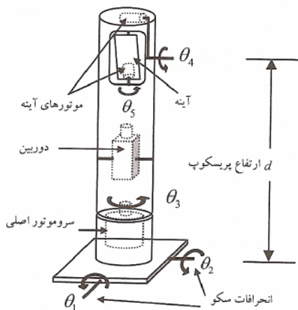
شکل ۱: ساختار پرسکوپ نوعی زیردریایی
