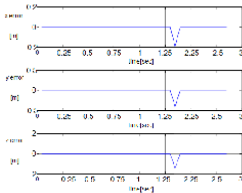
شکل 23: خطای ردیابی مجری نهایی با استفاده از روش شبه‌وارون ژاکوبی
