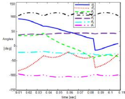
شکل 10: موقعیت نهایی مفاصل در حالت مقید
