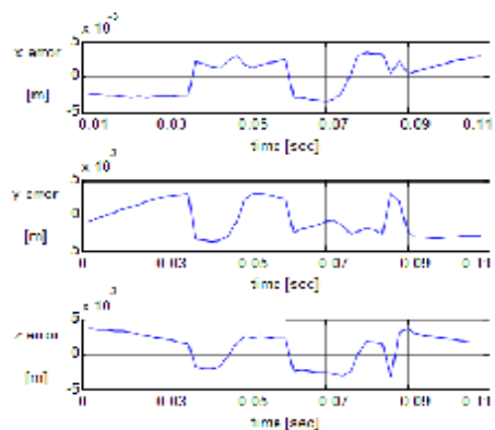
شکل 11: خطای ردیابی مجری نهایی
