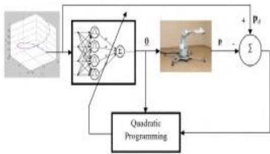
شکل 4: ساختار پیشنهادی بدون سیستم فازی برای جمع‌آوری داده‌های لازم جهت تشکیل سیستم فازی
