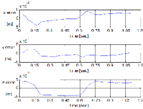
شکل 20: خطای ردیابی مجری نهایی با استفاده از روش پیشنهادی
