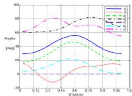
شکل 19: موقعیت نهایی مفاصل با استفاده از روش پیشنهادی
