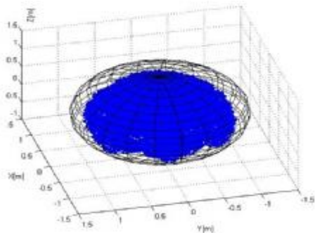
شکل 5: مجموعه‌ای از داده‌های فضای کاری ربات بازوی PA-10
