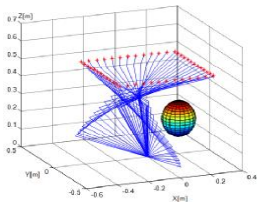
شکل 9: پیکربندی‌های نهایی ربات در حالت مقید
