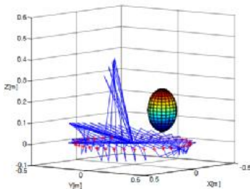
شکل 24: پیکربندی‌های ربات با استفاده از روش پیشنهادی
