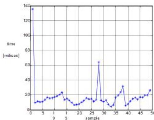
شکل 13: زمان اجرای محاسبات متناظر با نقاط مسیر مستطیلی
