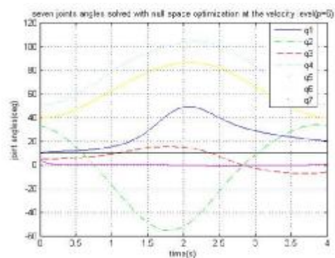
شکل 17: موقعیت نهایی مفاصل ربات [3]
