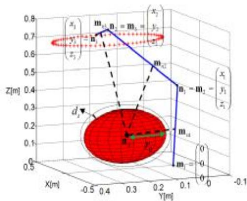
شکل 3: موقعیت نقاط روی بازوها و مانع نسبت به یکدیگر
