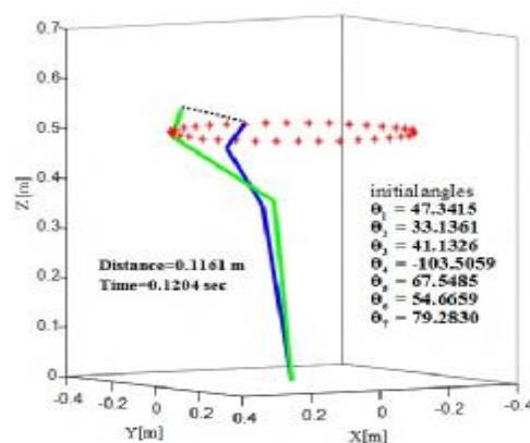
شکل 15: پیکربندی اولیه و نهایی ربات متناظر با اولین نقطه مطلوب با سیستم فازی
