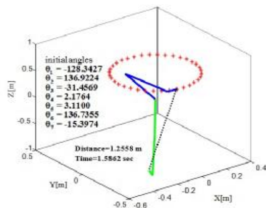
شکل 14: پیکربندی اولیه و نهایی ربات متناظر با اولین نقطه مطلوب بدون سیستم فازی
