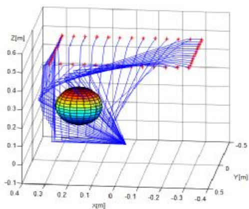
شکل 8: پیکربندی‌های نهایی ربات در حالت نامقید
