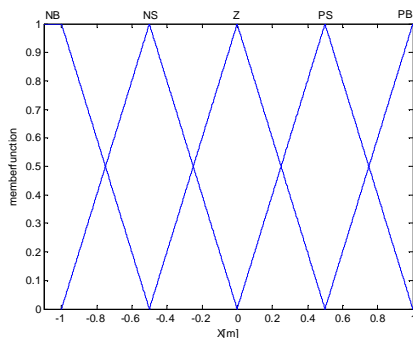
شکل 6: توابع عضویت ورودی X
