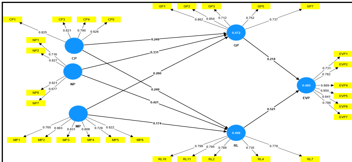
Fig. 3. PLS-SEM result.
