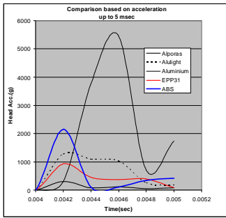
شکل ۶. شتاب کاهشی سر در ۵ میلی ثانیه از برخورد
