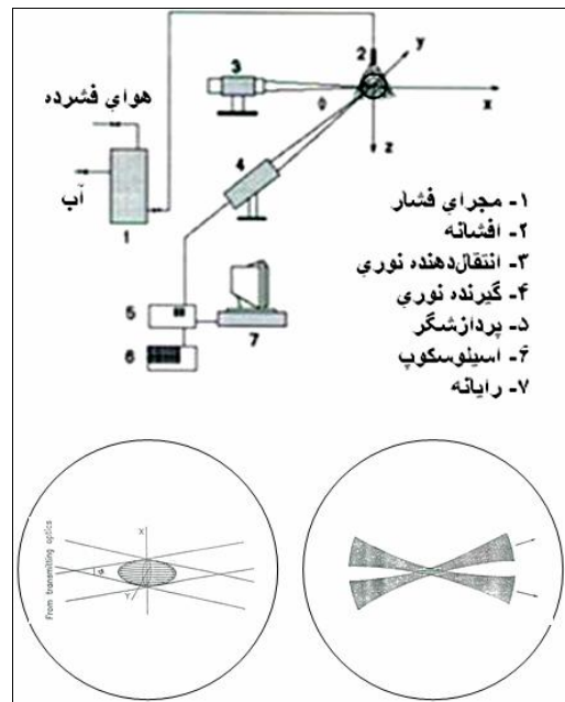
شکل ۳. چیدمان شماتیک سیستم PDA
