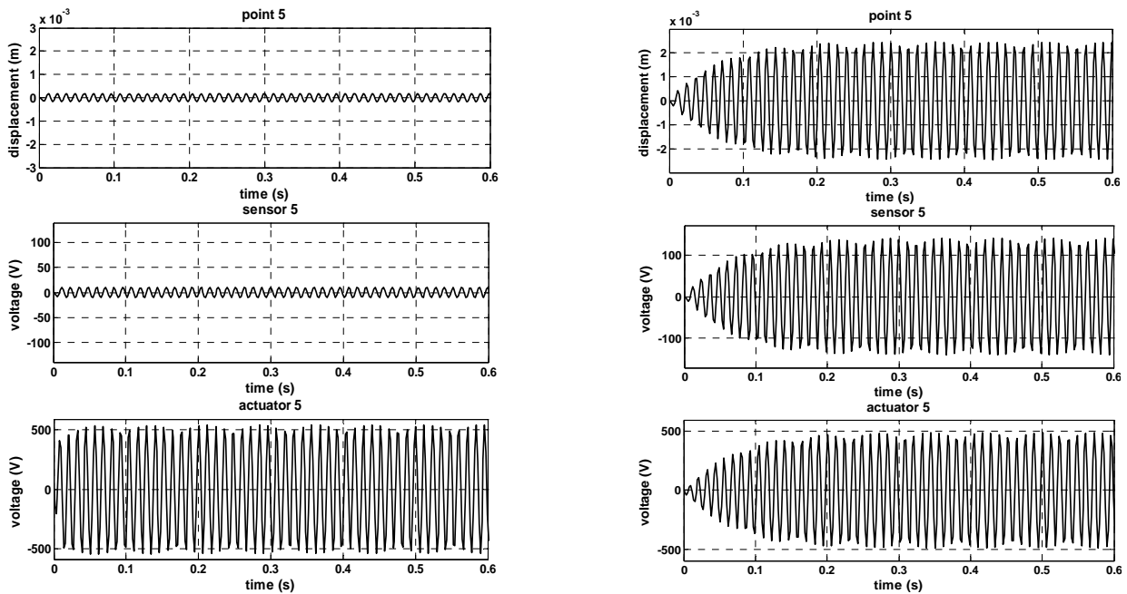
شکل ۸. نتایج وصله ۵ در حالت تشدید و ضرایب کنترل
