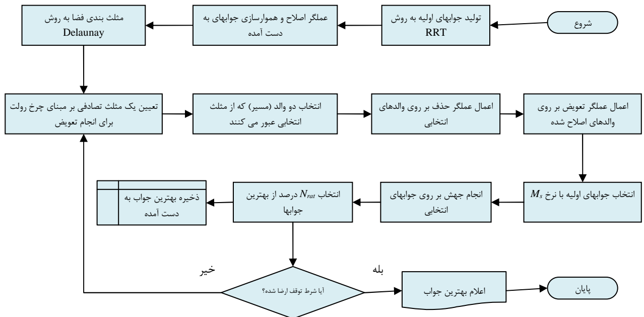
شکل ۱. فلوچارت روش پیشنهادی
