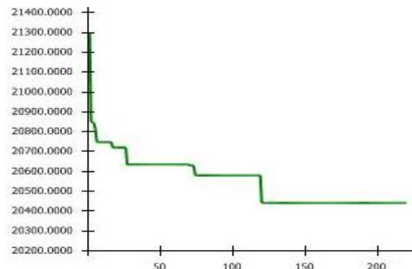
شکل ۳. نمودار بهینه‌سازی شبیه‌سازی سیستم تخصیص واگن‌های باری خالی توسط نرم‌افزار OptQuest
