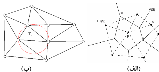
شکل ۷. الف) مثلث‌بندی دلونی (خط چین) به همراه دوگان و رونویسی آن؛ ب) نمایش خاصیت سوم مثلث‌بندی دلونی
